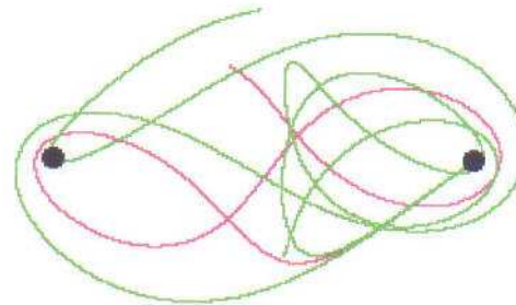
Sensibilité aux conditions initiales → Chaos
